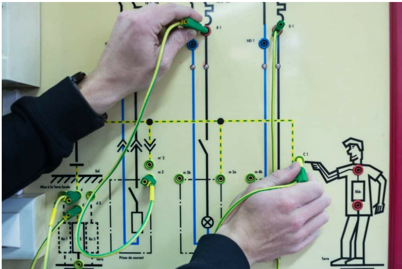
Platine de test de schéma de liaison à la terre à disposition des stagiaires.
