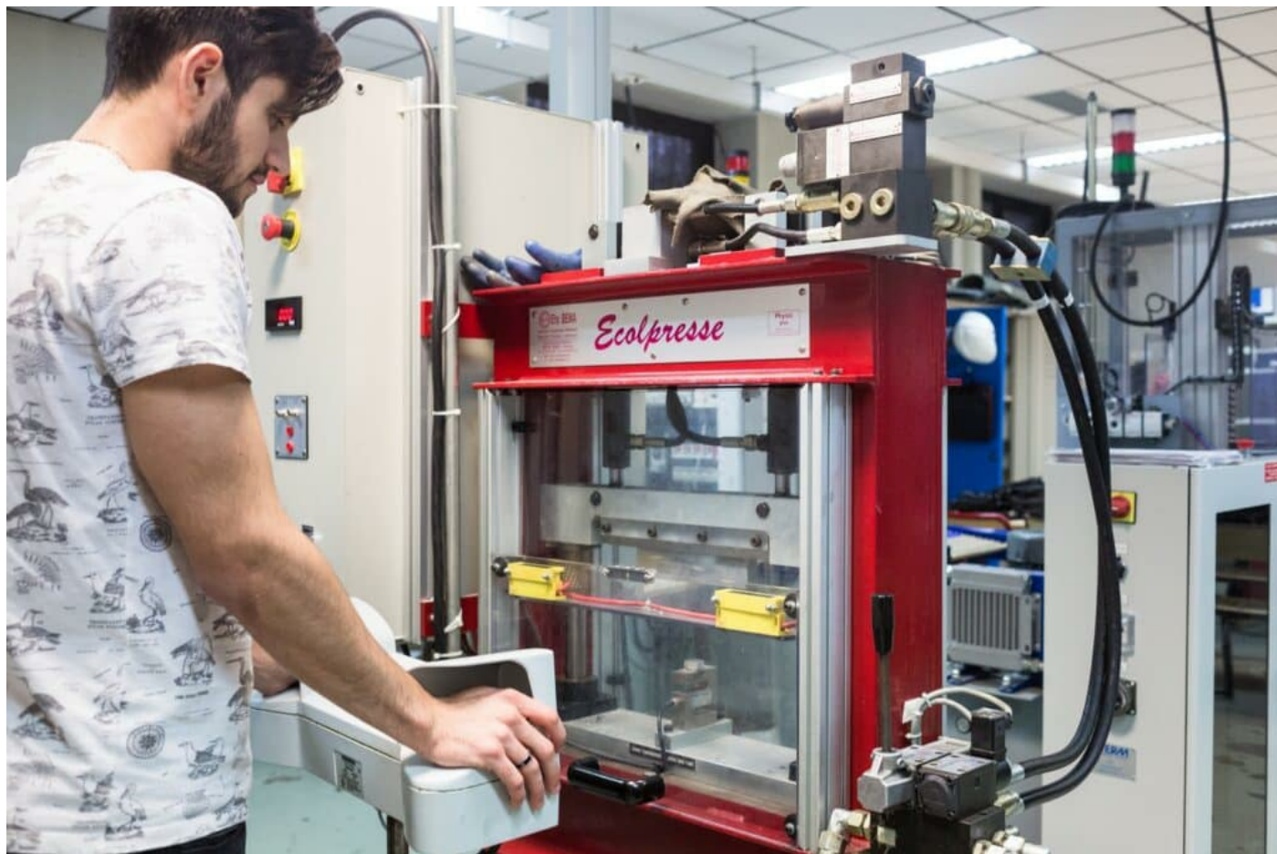
Mise en service du système de presse plieuse hydraulique Ecolpress par un stagiaire du BTS Maintenance des systèmes.
